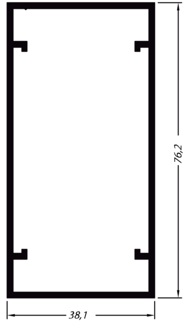
PC 003 P 6,300 kg/6m
