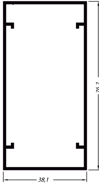
PC 003 4,800 kg/6m
