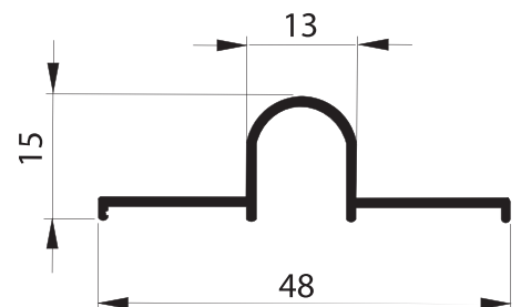
PC 007 1,500 kg/6m Inferior de Portão
