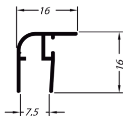
BX 226 BOX 0,900 kg/6m
