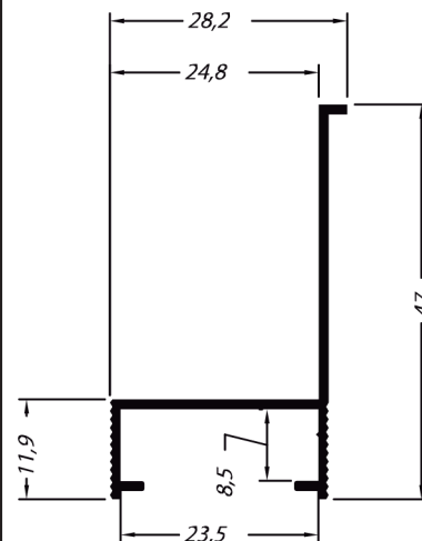
CM 151 1,750 kg/6m
