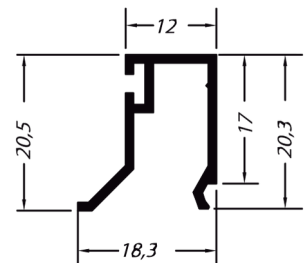
AL 27 1,000 kg/6m
