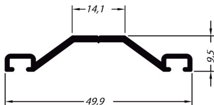
DS 1102 1,700 kg/6m
