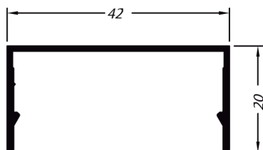
FC 013 1,500 kg/6m
