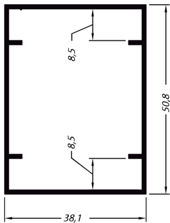
PC 010 6,000 kg/6m
