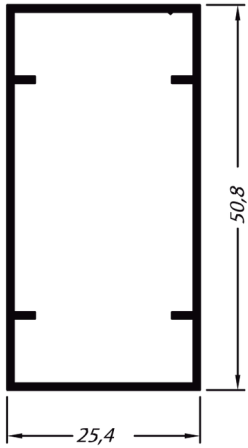
PC 002 2,400 kg/6m
