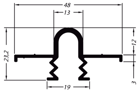
PC 007 1,500 kg/6m Inferior de Portão
