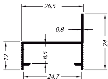
CM 200 0,900 kg/6m
